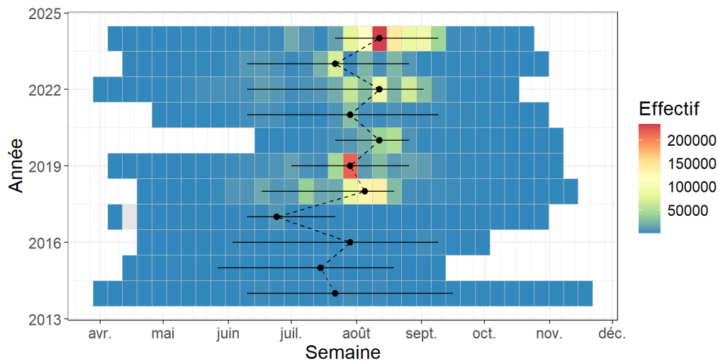
FIGURE 27 – Rythmes migratoires des anguilles capturées dans les passes pièges du barrage de Poses - Amfreville-sous-les-Monts.
