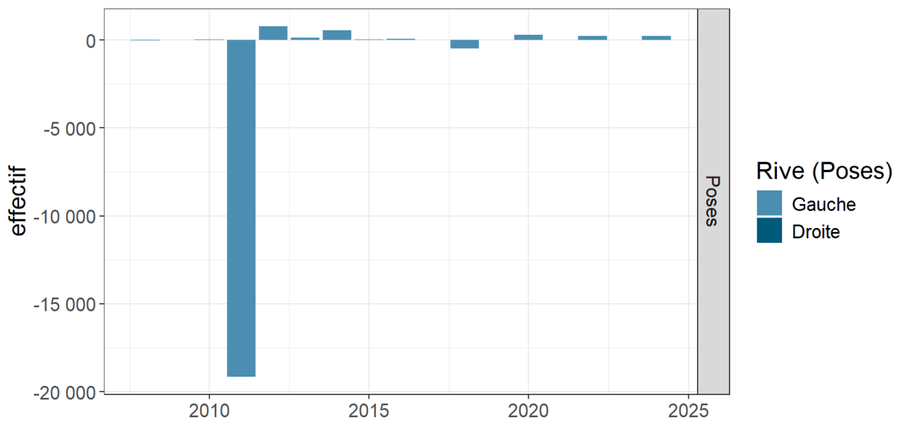
FIGURE 37 – Evolution interannuelle des effectifs de lamproies fluviatiles recensés sur les STACOMI du bassin Seine.
