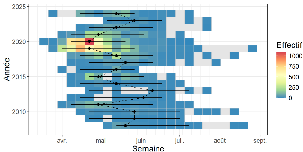
FIGURE 20 – Rythmes migratoires des aloses au barrage de Poses - Amfreville-sous-les-Monts.
