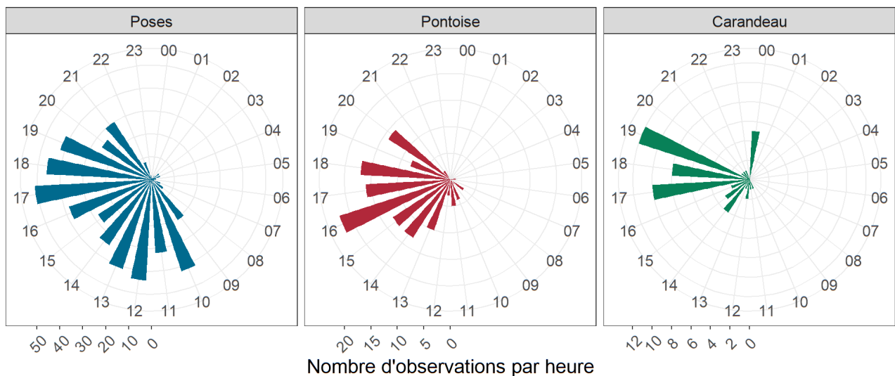
FIGURE 22 – Horaires de migration des aloses en 2024
