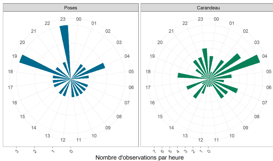
FIGURE 35 – Horaires de migration des anguilles argentées en 2024
