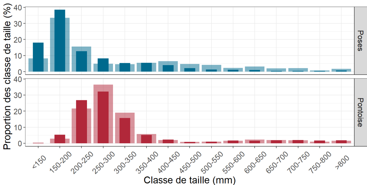
FIGURE 31 – Distribution de tailles des anguilles jaunes mesurées aux stations de Poses et de Pontoise.
