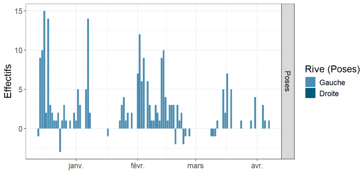
FIGURE 36 – Effectifs journaliers des lamproies fluviatiles recensés sur les STACOMI du bassin Seine.
