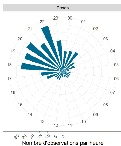
FIGURE 39 – Horaires de migration des lamproies fluviatiles en 2024
