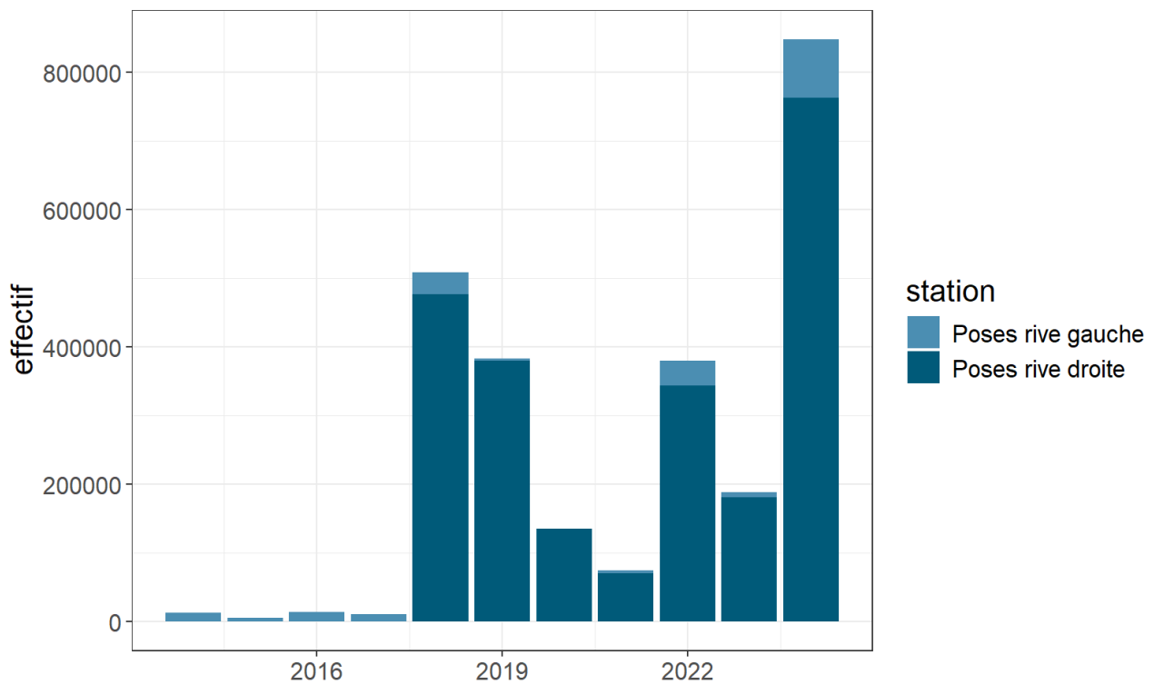
FIGURE 26 – Evolution interannuelle des effectifs des anguilles capturées dans les passes pièges au barrage de Poses - Amfreville-sous-les-Monts
