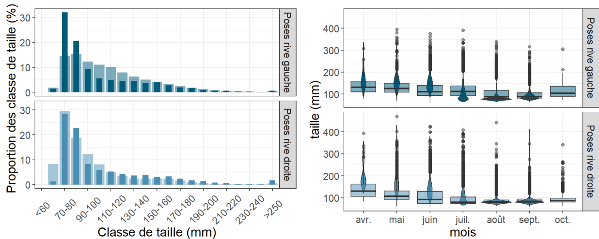
FIGURE 27 – Représentation des tailles des Anguilles capturées dans les passes-pièges du barrage de Poses - Amfreville-sous-les-Monts. Les tailles historiques sont présentées en transparence sur les deux graphiques
