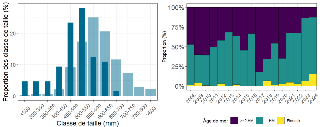
FIGURE 63 – Représentation des tailles et des âges de mer des truites de mer observées en vidéocompage au barrage de Poses - Amfreville-sous-les-Monts. Les tailles historiques sont présentées en transparence sur le graphique de gauche.
