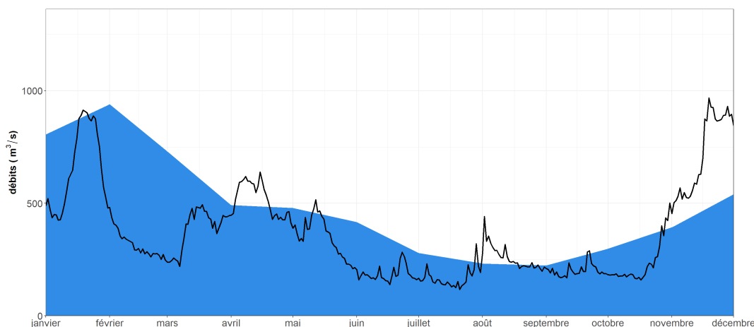
FIGURE 2 – Régime hydrologique de la Seine à Vernon, la moyenne interannuelle des dix années précédentes (2012 à 2022) est représentée en bleu, les débits journaliers de l'année sont présentés en noir
