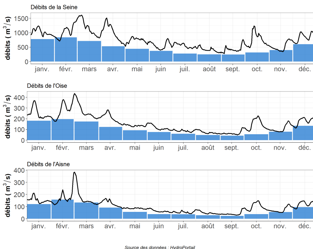
FIGURE 2 – Régime hydrologique de la Seine, de l'Oise et de l'Aisne, le débit moyen mensuel est représentée en bleu, les débits journaliers de l'année sont présentés en noir
