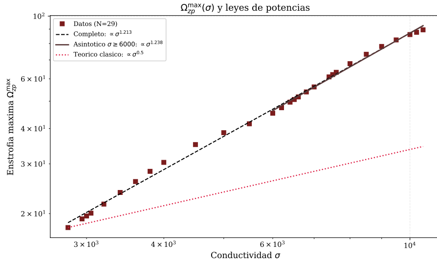
Figura 6.8: \Omega_{zp}^{\max}(\sigma) en escala log-log, con los dos ajustes empíricos (completo y asintótico) y el escalamiento \sigma^{1/2} de una lámina de corriente Sweet–Parker única. La pendiente empírica ( \alpha \approx 1,22 ) es marcadamente más pronunciada que ese piso, lo que indica una superficie disipativa que crece más rápido que una única lámina.
