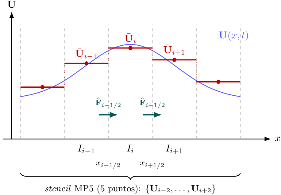
Figura 4.1: Representación esquemática de la discretización espacial bajo el formalismo de volúmenes finitos unidimensionales. Se ilustra la transición desde el estado continuo del plasma U(x, t) hacia su representación discreta mediante promedios espaciales \bar{U}_i^n confinados en los volúmenes de control I_i . La evolución temporal del sistema está dictada por los flujos numéricos [REV: de interfaz] ([REV: CAMBIAR INTERFACIAL POR INTERFAZ O DE INTERFAZ]) interfasiales \hat{F}_{i\pm 1/2} , evaluados en las fronteras espaciales x_{i\pm 1/2} , los cuales garantizan la conservación estricta de las variables de estado durante el intercambio físico entre celdas adyacentes.
