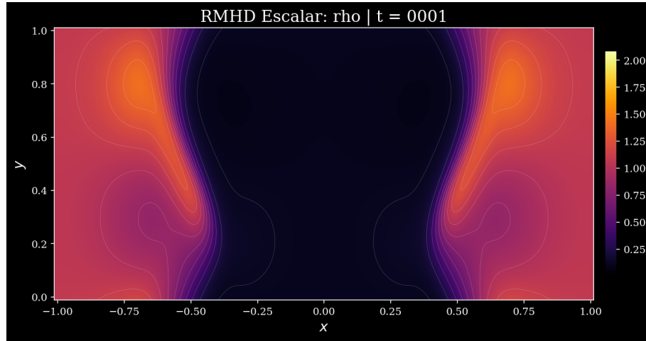
(b) Distribución de densidad \rho(x,y) con contornos isóbaros superpuestos. Se observa nítidamente la región interior de baja densidad ( \rho \simeq \rho_{lo} , |x| < 0,5 ) embebida en el ambiente externo de alta densidad ( \rho \simeq \rho_{up} , |x| > 0,5 ), consistente con la ventana hiperbólica prescrita por la Ec. (5.3). Las modulaciones longitudinales tempranamente visibles en las interfaces reflejan la incipiente respuesta vortical del fluido a la perturbación inyectada.
