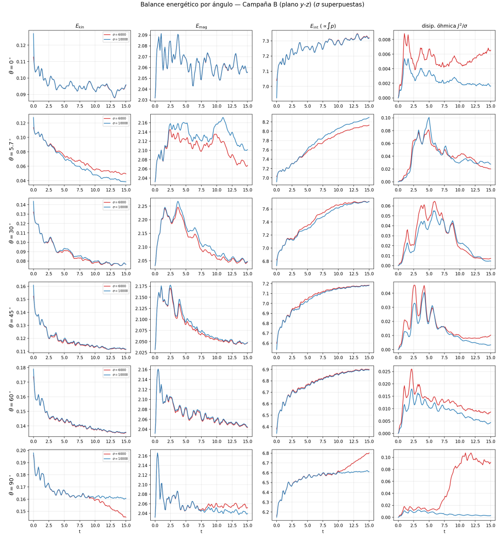
Figura 6.28: Campaña B (plano y - z ): balance energético por ángulo. Filas = \theta ; columnas = E_{kin} , E_{mag} , E_{int} (calor) y tasa de disipación óhmica \int J^2/\sigma . En rojo \sigma = 6000 , en azul \sigma = 10000 .
