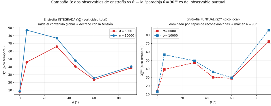
Figura 6.21: Campaña B (plano y-z ): enstrofia de perturbación frente al ángulo \theta , en dos observables. Izquierda : enstrofia integrada \Omega_{zp}^{int} (contenido total de vorticidad), máxima a \theta bajo y decreciente con la tensión. Derecha : máximo puntual \Omega_{zp}^{max} , dominado por capas de reconexión finas y máximo en \theta = 90^\circ . La discrepancia muestra que la “paradoja” de \theta = 90^\circ es un efecto del observable, no de la física de tensión. ( \sigma = 6000 , CFL=0,04; \sigma = 10000 , CFL=0,02.)
