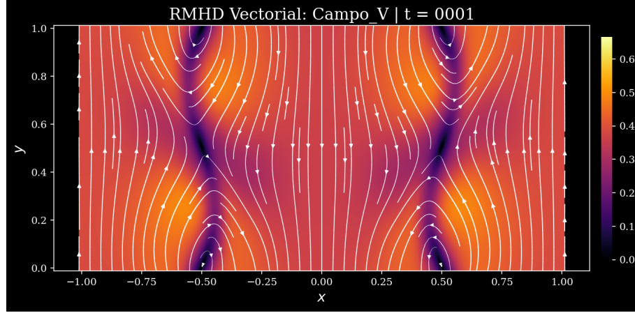
(a) Campo vectorial de velocidad: líneas de corriente superpuestas al mapa de color de la magnitud |\mathbf{V}(x,y)| . Se aprecian las dos capas de cizalladura simétricas localizadas en x = \pm 0,5 (regiones oscuras de baja magnitud), el cambio de signo de V_y a través de cada interfaz, y la modulación senoidal transversal de período L_y introducida por la perturbación de la Ec. (5.2), responsable de la semilla del modo inestable dominante.
