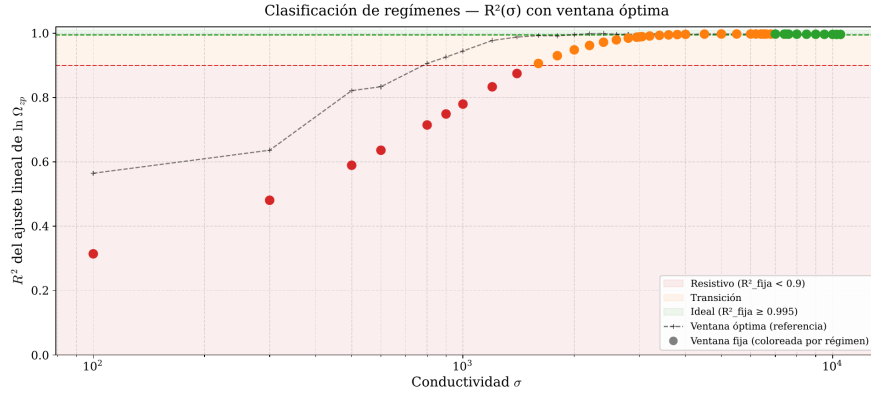
Figura 6.8: Construcción de la zona de transición: coeficiente R^2_{\text{fija}} del ajuste lineal de \ln \Omega_{zp}(t) frente a \sigma . Los umbrales clasifican cada simulación en régimen resistivo ( R^2 < 0,90 , rojo), transición ( 0,90 \leq R^2 < 0,995 , naranja) o ideal ( R^2 \geq 0,995 , verde), delimitando la banda \sigma \in [1400, 7000] donde se localiza \sigma_{\text{crit}} . La línea discontinua es el R^2 con ventana óptima, como referencia.
