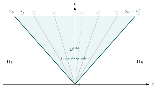
Estados U_L, U_R reconstruidos (MP5) en la interfaz a t = t^n
