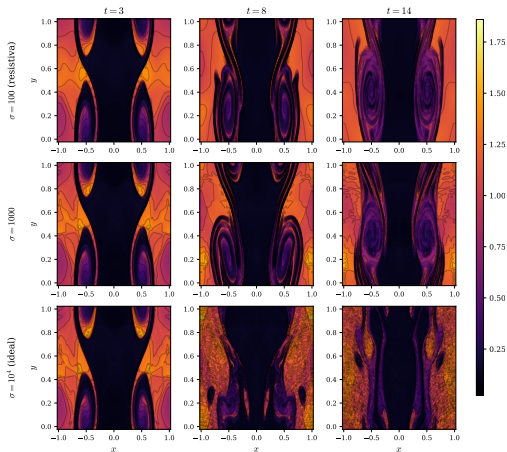
Variación de conductividad — densidad \rho
