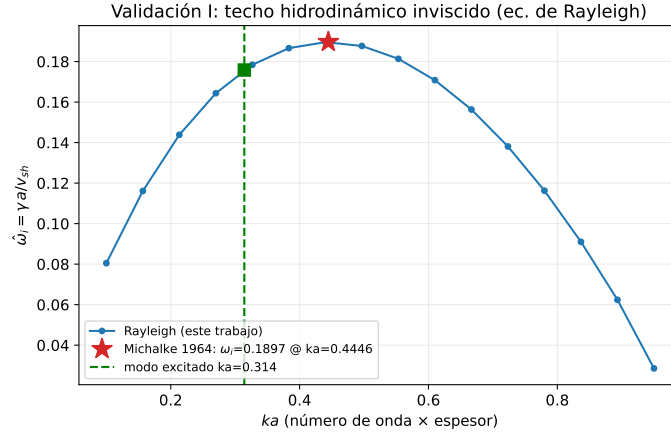
Figura 6.14: Validación del solver de autovalores. Tasa de crecimiento adimensional \hat{\omega}_i(ka) de la ecuación de Rayleigh (este trabajo) frente al valor de Michalke [22]. El cuadrado verde marca el modo excitado en las simulaciones.
