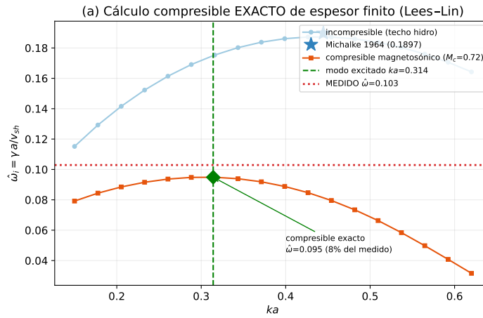
Figura 6.16: Cálculo compresible exacto de espesor finito (Lees-Lin), validado contra Michalke [22] en el límite incompresible. La curva magnetosónica pica en ka \simeq 0,32 con \hat{\omega} = 0,095 , justo en el modo excitado; el valor medido (0,103) coincide dentro del 8%.
