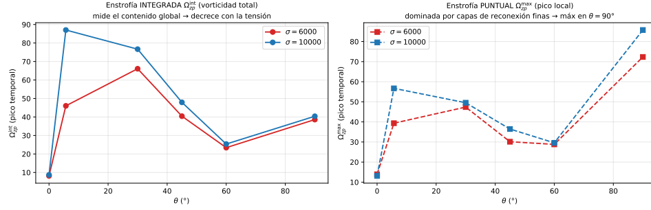
Figura 6.21: Campaña B (plano y-z ): enstrofia de perturbación frente al ángulo \theta , en dos observables. Izquierda : enstrofia integrada \Omega_{zp}^{int} (contenido total de vorticidad), máxima a \theta bajo y decreciente con la tensión. Derecha : máximo puntual \Omega_{zp}^{max} , dominado por capas de reconexión finas y máximo en \theta = 90^\circ . La discrepancia muestra que la “paradoja” de \theta = 90^\circ es un efecto del observable, no de la física de tensión. ( \sigma = 6000 , CFL= 0,04; \sigma = 10000 , CFL= 0,02.)
