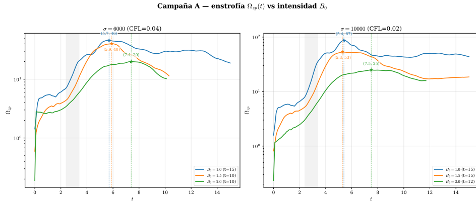
Figura 6.19: Campaña A (intensidad): enstrofia de perturbación \Omega_{zp}(t) para B_0 = 1,0, 1,5, 2,0 a \sigma = 6000 (CFL=0,04) y \sigma = 10000 (CFL=0,02). El pico se atenúa y se retrasa al aumentar B_0 .
