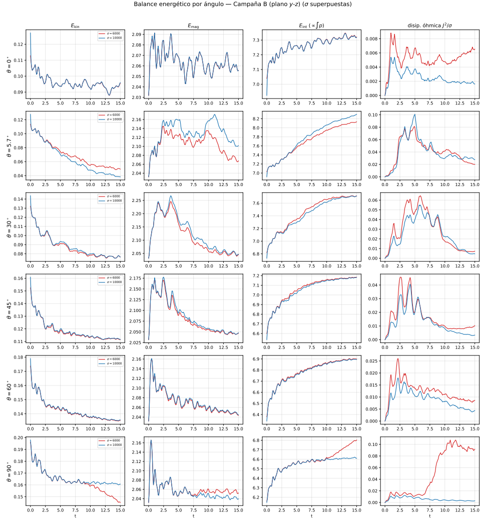
Figura 6.28: Campaña B (plano y - z ): balance energético por ángulo. Filas = \theta ; columnas = E_{kin} , E_{mag} , E_{int} (calor) y tasa de disipación óhmica \int J^2/\sigma . En rojo \sigma = 6000 , en azul \sigma = 10000 .
