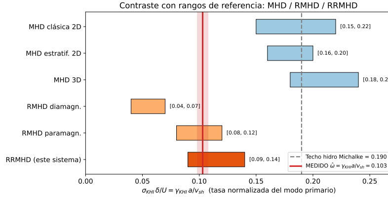
Figura 6.18: Tasa medida ( \hat{\omega} = 0,103 , línea roja) frente a los rangos de referencia de \sigma_{KHI} . El techo hidrodinámico (gris, 0,190) cae en el bloque clásico MHD; el valor medido cae en el bloque relativista (RMHD/RRMHD), confirmando la supresión relativista–compresible. Las filas de polarización magnética corresponden a Pimentel y Lora-Clavijo [34].
