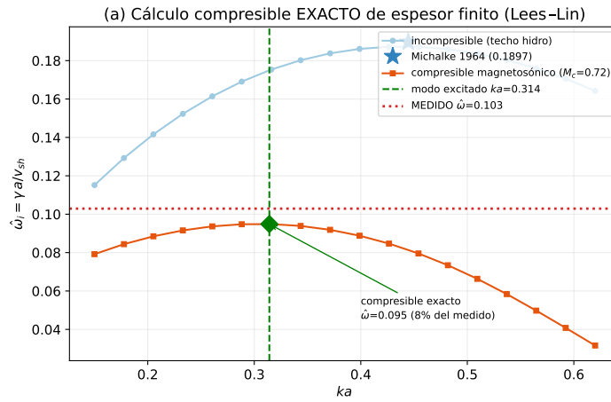
Figura 6.16: Cálculo compresible exacto de espesor finito (Lees–Lin), validado contra Michalke [21] en el límite incompresible. La curva magnetosónica pica en ka \simeq 0,32 con \hat{\omega} = 0,095 , justo en el modo excitado; el valor medido (0,103) coincide dentro del 8%.
