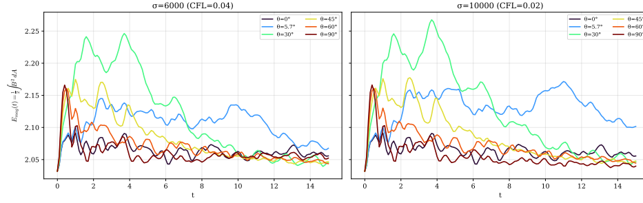
Figura 6.22: Campaña B: energía magnética E_{mag}(t) = \frac{1}{2} \int B^2 dA por ángulo; sus valles se acoplan con los picos de enstrofia.
