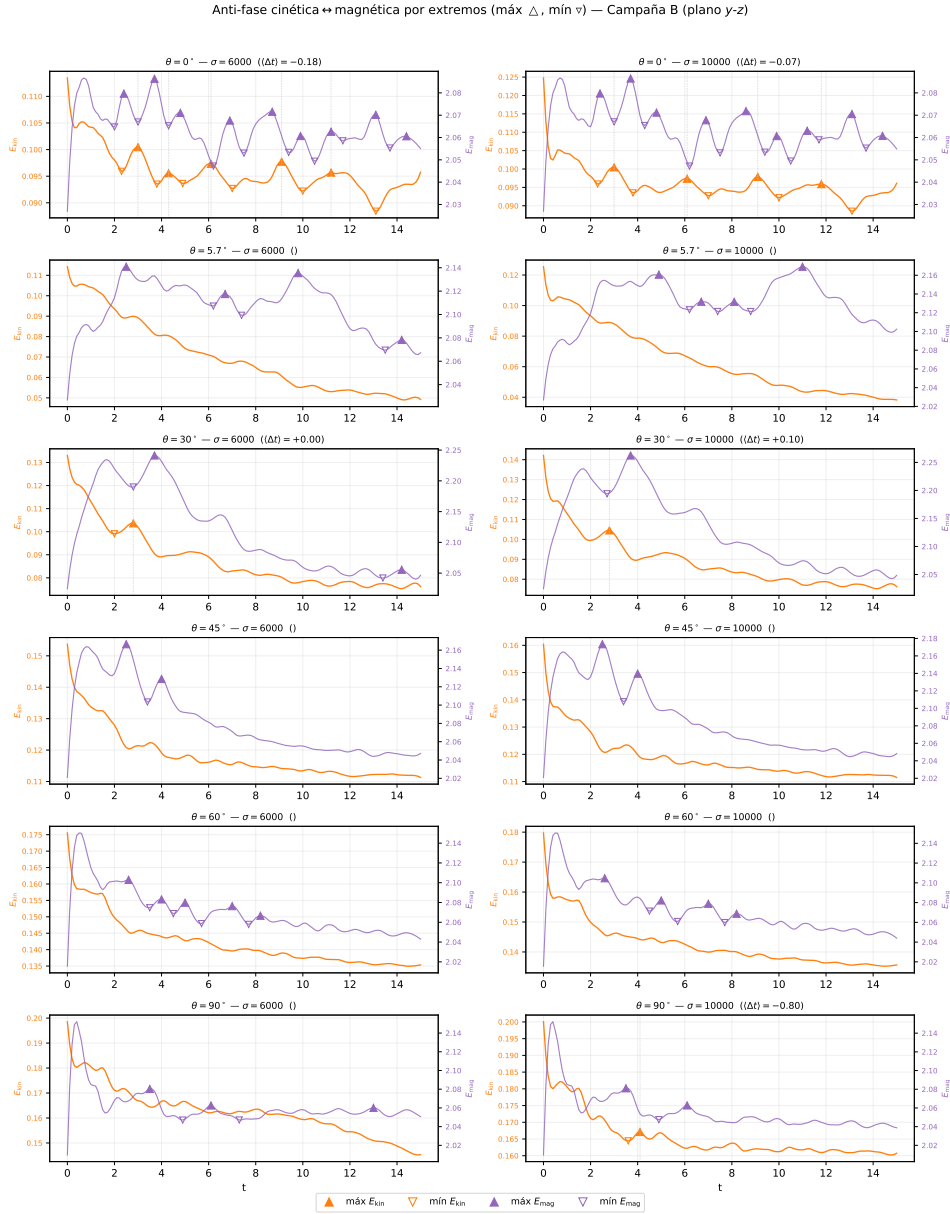
Figura 6.24: Campaña B: energía cinética E_{kin} (naranja) y magnética E_{mag} (morado) con sus extremos locales (máximos \Delta , mínimos \nabla ) por cruce-cero de la derivada, para cada ángulo y conductividad. Los máximos de una coinciden con los mínimos de la otra: el intercambio cinético↔magnético procede por ciclos repetidos en anti-fase. [REV: hay que ver bien por que veo maximos y minimos locales no marcados]
