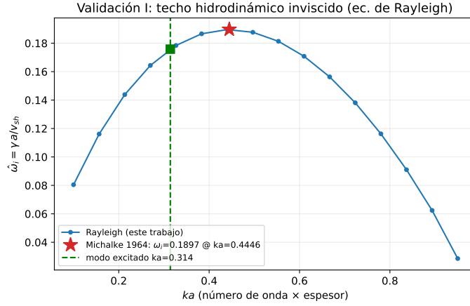
Figura 6.14: Validación del solver de autovalores. Tasa de crecimiento adimensional \hat{\omega}_i(ka) de la ecuación de Rayleigh (este trabajo) frente al valor de Michalke [21]. El cuadrado verde marca el modo excitado en las simulaciones.
