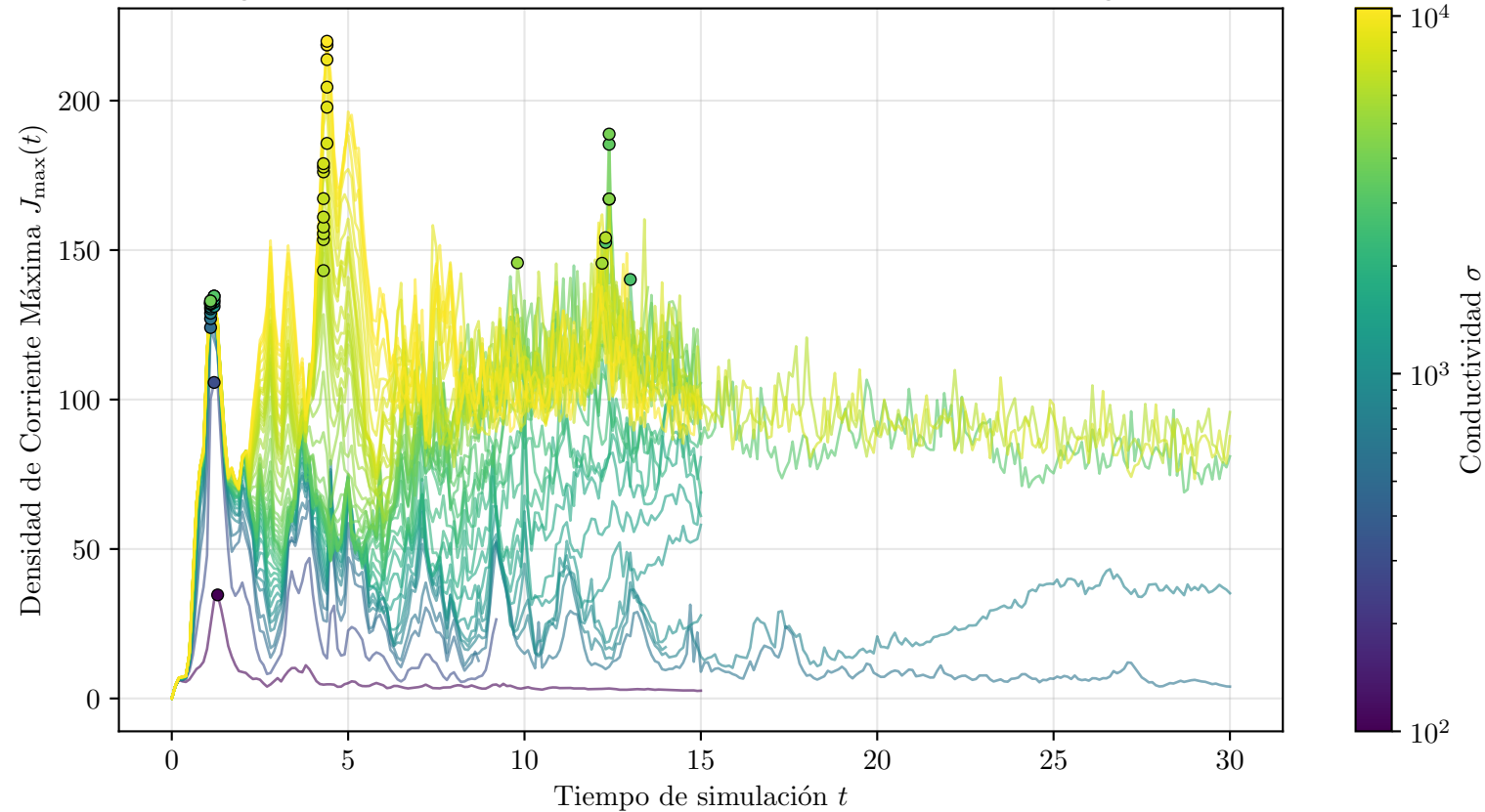
Diagnóstico de topometría de corriente: Localización de picos globales
