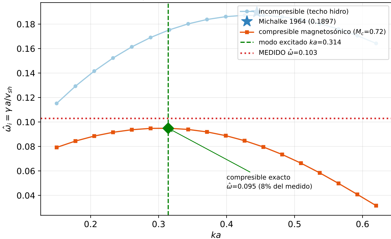
(a) Cálculo compresible EXACTO de espesor finito (Lees-Lin)
