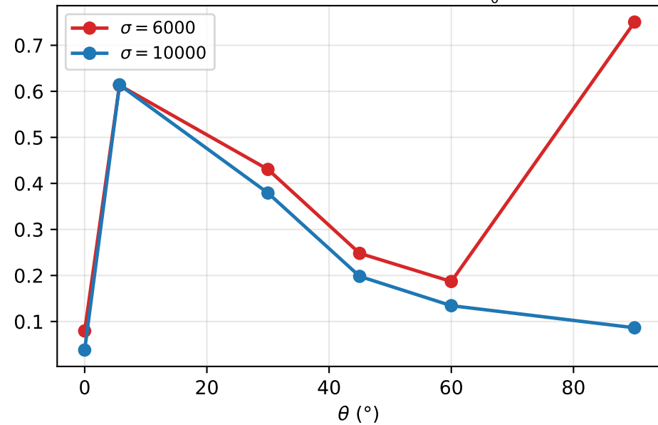
Disipación óhmica acumulada \int_0^{t_f} \frac{j^2}{\sigma} dt
