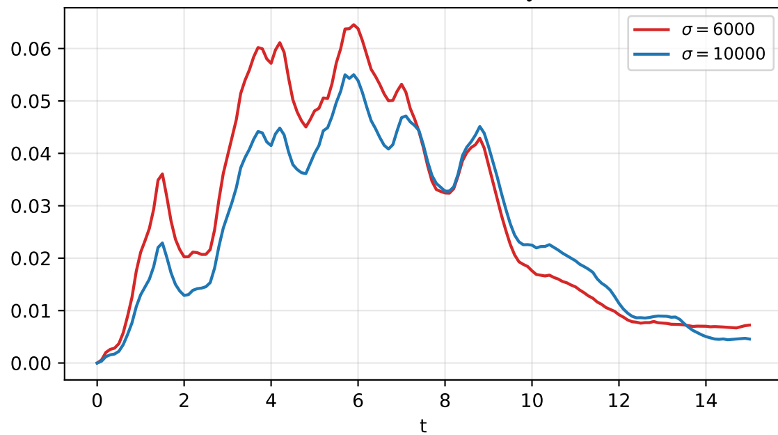
Tasa de disipación óhmica \int j^2 / \sigma
