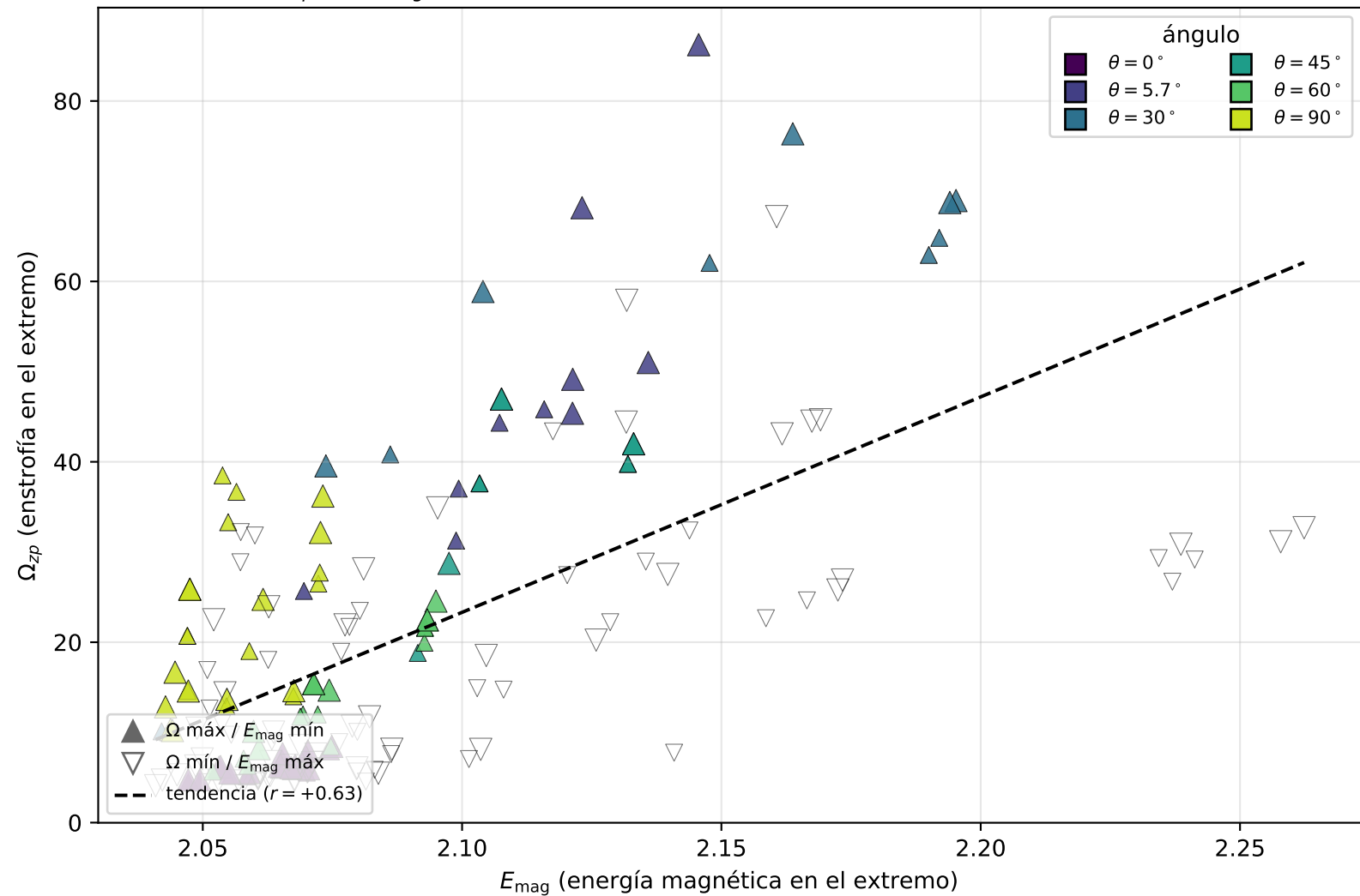
\Omega_{zp} vs E_{\text{mag}} en los extremos (máx y mín) — Campaña B (plano y-z)
