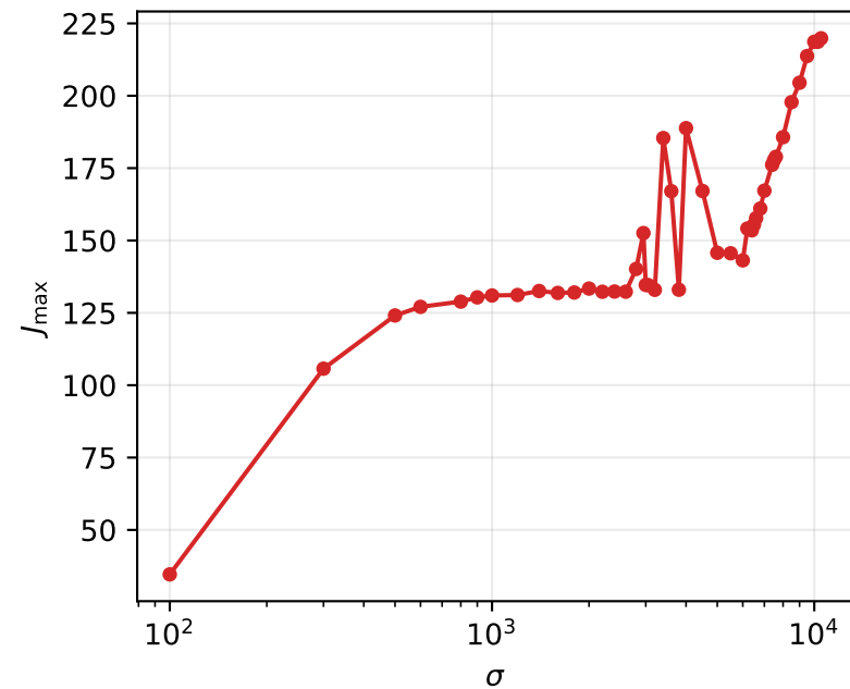
(a) Corriente máxima J_{\max}(\sigma)
