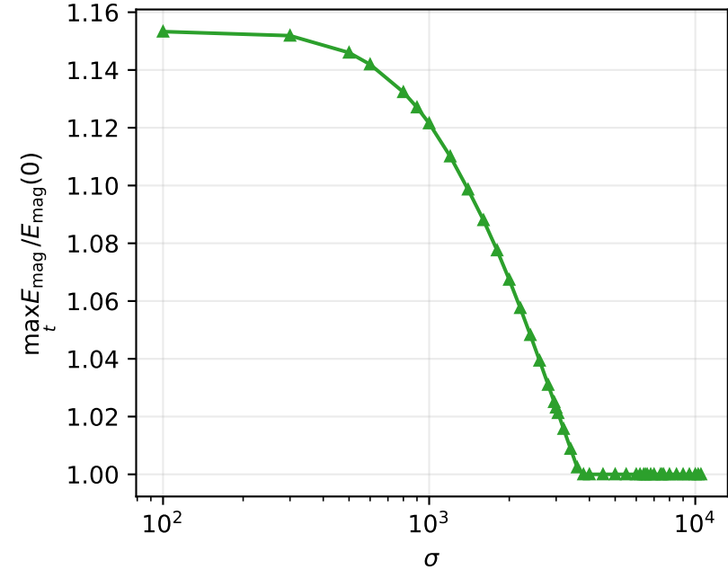
(c) Amplificación de energía magnética
