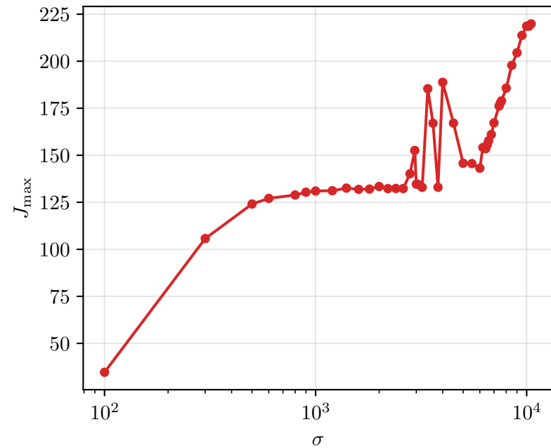
(a) Corriente máxima J_{\max}(\sigma) [Global/Ciego]
