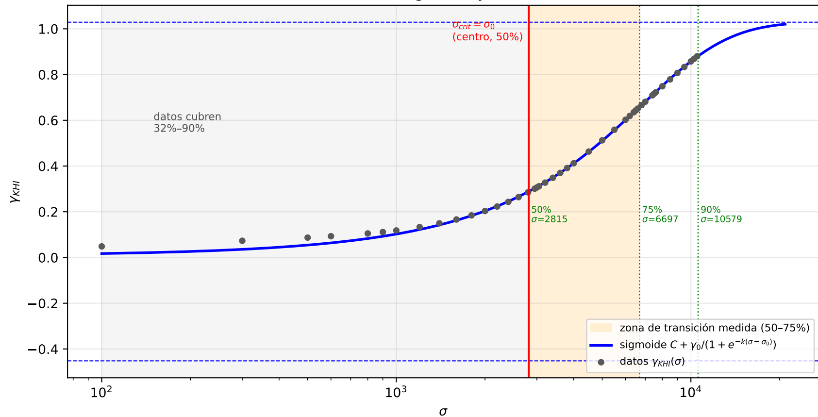
Forma de la transición: sigmoide y fracciones del ascenso
