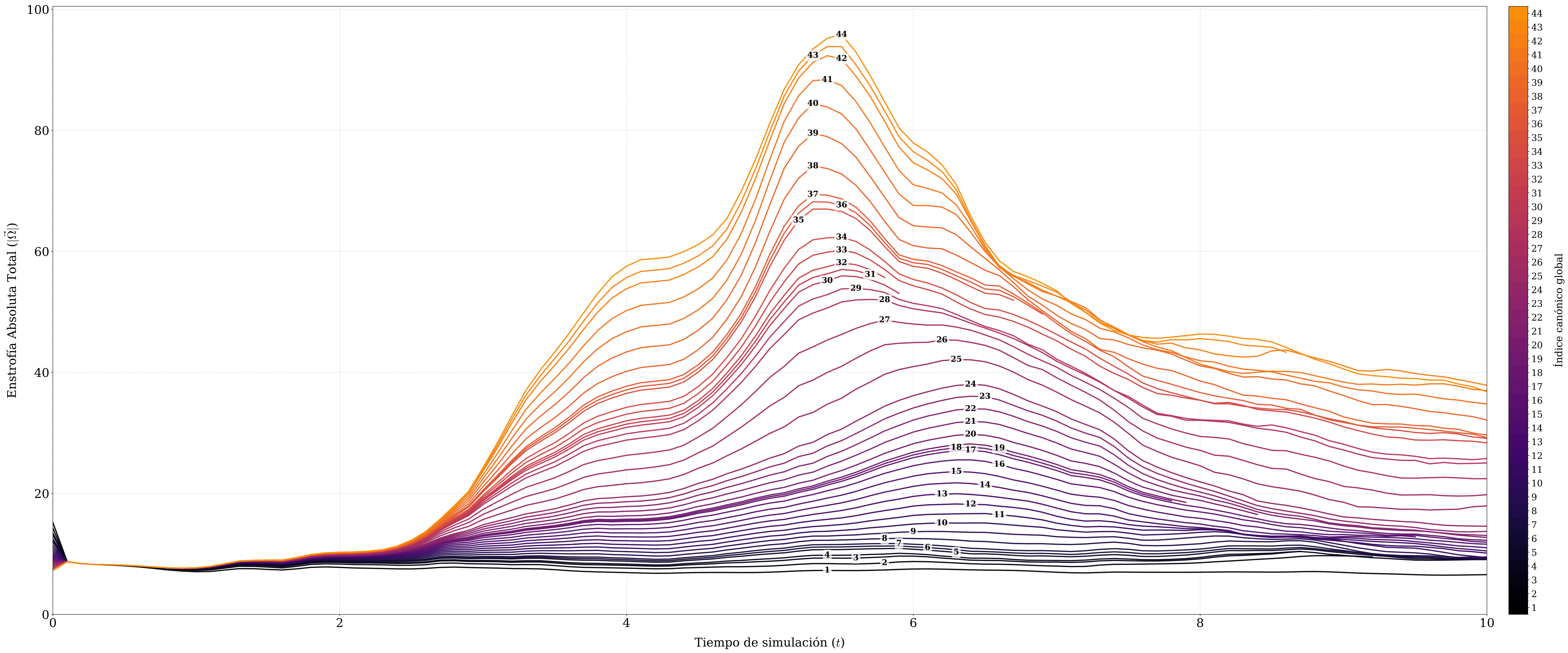
RRMHD-KHI: Enstrofía Absoluta Total (supervivencia t > 3.0 , anotación t \in [5.0, 9.0] )
