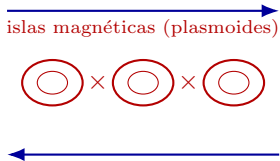
(b) modo tearing : cadena de islas
