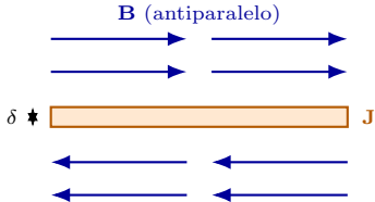
(a) lámina de corriente
