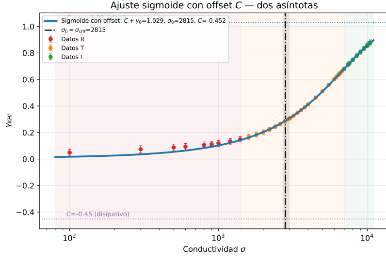
Figura 6.5: Ajuste sigmoide de la tasa de crecimiento efectiva \gamma_{\text{KHI}} frente a la conductividad \sigma . Las bandas indican los regímenes resistivo, transitorio e ideal; la línea vertical marca \sigma_{\text{crit}} (punto de inflexión) y la banda gris su incertidumbre. Las asíntotas del modelo son la superior C + \gamma_0 \simeq 1,03 (casi ideal) y la inferior C \simeq -0,45 ( offset ).
