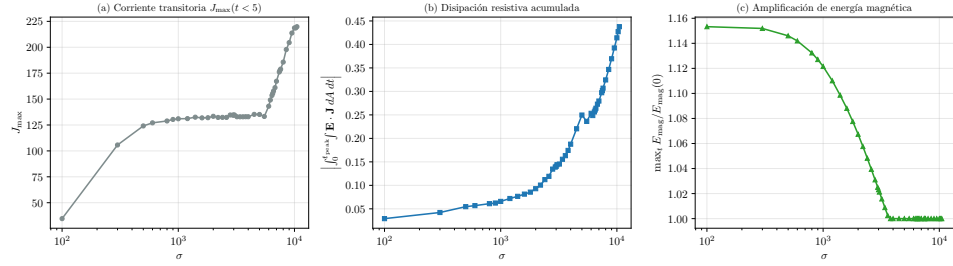
Figura 6.13: Variables electromagnéticas globales frente al parámetro de conductividad \sigma . (a) Densidad de corriente máxima J_{\max} evaluada estrictamente durante el régimen transitorio inicial ( t < 5,0 ). Las oscilaciones paramétricas a bajos \sigma no corresponden a reconexión magnética turbulenta, sino a los gradientes máximos generados por la relajación numérica de la discontinuidad inicial (problema de Riemann). Su eventual estabilización evidencia el umbral paramétrico de transición donde la difusividad física del plasma supera el error de truncamiento de la malla. (b) Trabajo electromagnético (disipación de Joule) acumulado hasta el tiempo físico de saturación t_{\text{peak}} . (c) Amplificación de la energía magnética propia (comóvil) alcanzada en la saturación.
