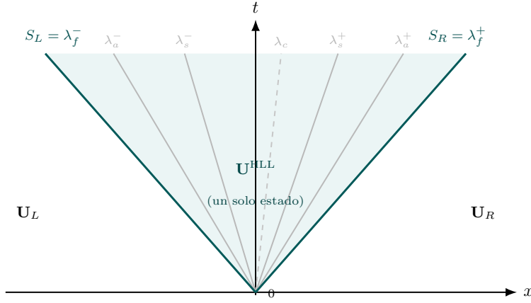
Estados \mathbf{U}_L, \mathbf{U}_R reconstruidos (MP5) en la interfaz a t = t^n
