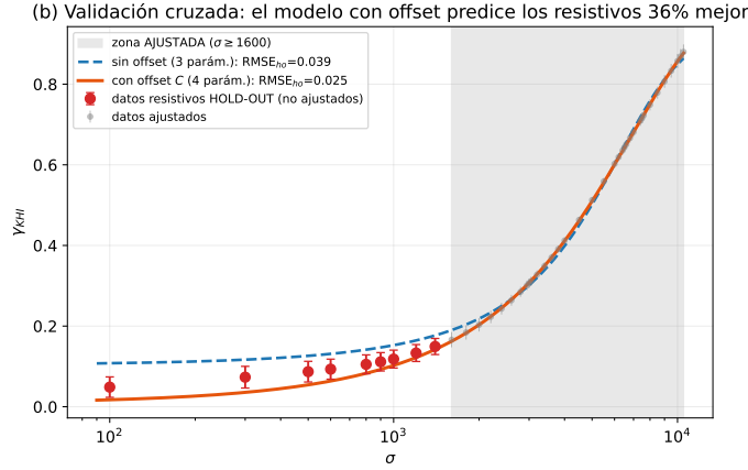
Figura 6.7: Validación cruzada. Ajuste en \sigma \geq 1600 (zona gris); los puntos rojos ( \sigma < 1600 ) son hold-out . El modelo con offset predice los resistivos retenidos un 36 % mejor que el de tres parámetros.
