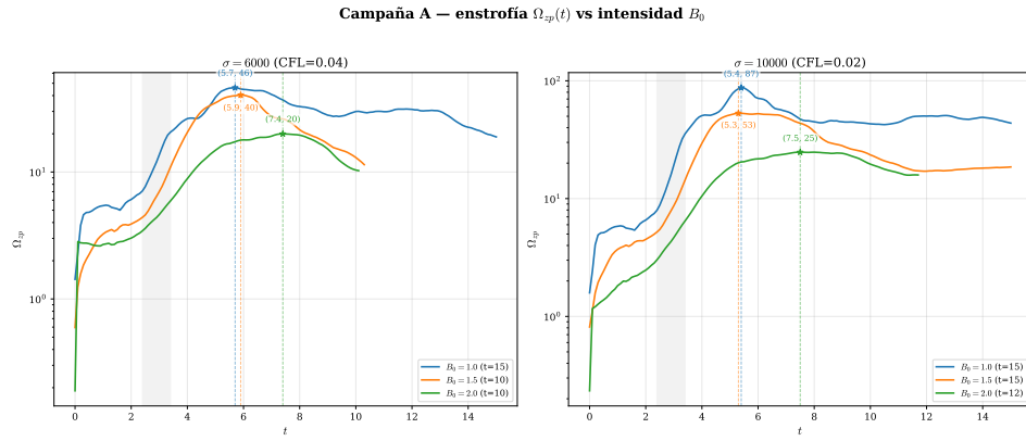
Figura 6.21: Campaña A (intensidad): enstrofia de perturbación \Omega_{zp}(t) para B_0 = 1,0, 1,5, 2,0 a \sigma = 6000 (CFL= 0,04) y \sigma = 10000 (CFL= 0,02). El pico se atenúa y se retrasa al aumentar B_0 .
