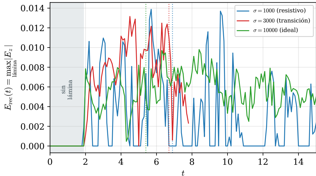
(b) Campo de reconexión en la lámina
