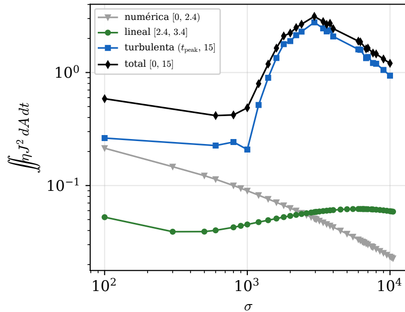
(b) Disipación resistiva acumulada por ventana
