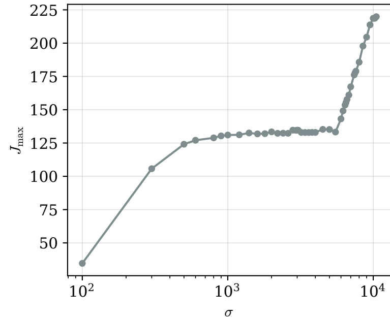
(a) Corriente transitoria J_{\max}(t < 5)
