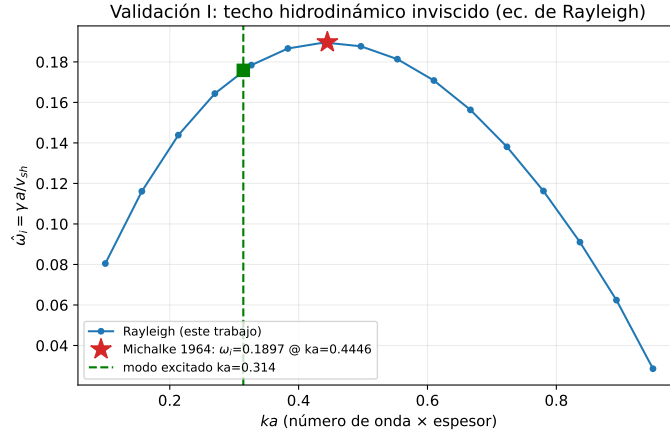
Figura 6.11: Validación del solver de autovalores. Tasa de crecimiento adimensional \hat{\omega}_i(ka) de la ecuación de Rayleigh (este trabajo) frente al valor de Michalke [38]. El cuadrado verde marca el modo excitado en las simulaciones.
