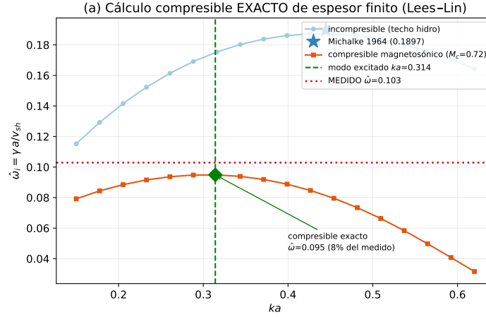
Figura 6.13: Cálculo compresible exacto de espesor finito (Lees-Lin), validado contra Michalke [38] en el límite incompresible. La curva magnetosónica pica en ka \simeq 0,32 con \hat{\omega} = 0,095 , justo en el modo excitado; el valor medido (0,103) coincide dentro del 8 %.
