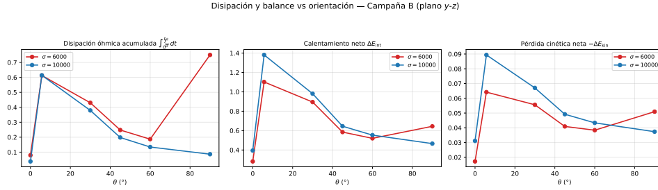
Figura 6.30: Campaña B: disipación óhmica acumulada, calentamiento neto \Delta E_{int} y pérdida cinética neta -\Delta E_{kin} en función del ángulo \theta , para ambas conductividades.
