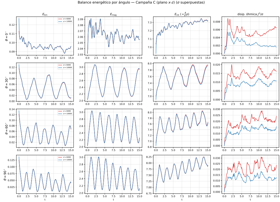
Figura 6.31: Campaña C (plano x - z ): balance energético por ángulo (filas = \theta ; columnas = E_{kin} , E_{mag} , E_{int} , disipación óhmica). En rojo \sigma = 6000 , en azul \sigma = 10000 .
