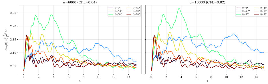
Figura 6.22: Campaña B: energía magnética E_{\text{mag}}(t) = \frac{1}{2} \int B^2 dA por ángulo; sus valles se acoplan con los picos de enstrofia.
