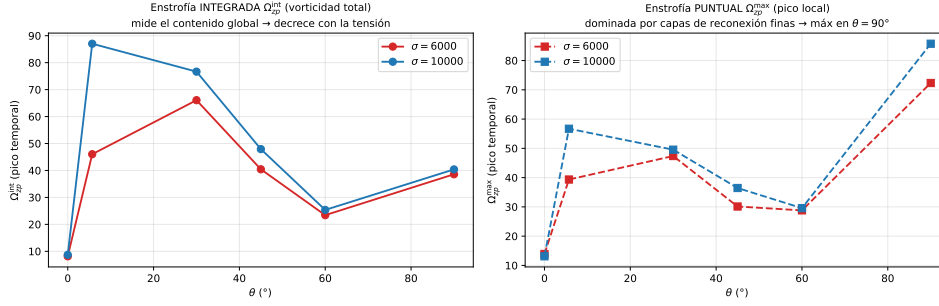
Figura 6.21: Campaña B (plano y-z ): enstrofia de perturbación frente al ángulo \theta , en dos observables. Izquierda : enstrofia integrada \Omega_{zp}^{int} (contenido total de vorticidad), máxima a \theta bajo y decreciente con la tensión. Derecha : máximo puntual \Omega_{zp}^{max} , dominado por capas de reconexión finas y máximo en \theta = 90^\circ . La discrepancia muestra que la “paradoja” de \theta = 90^\circ es un efecto del observable, no de la física de tensión. ( \sigma = 6000 , CFL=0,04; \sigma = 10000 , CFL= 0,02.)
