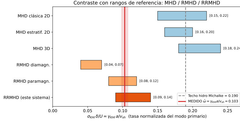
Figura 6.18: [REV: Comparación de la tasa de crecimiento normalizada del modo primario, \hat{\omega} = \gamma_{KHI} a/v_{sh} , con rangos de referencia reportados para configuraciones MHD, RMHD y RRMHD. La línea roja indica el valor medido en este trabajo, \hat{\omega} = 0,103 , mientras que la línea gris marca el límite hidrodinámico de referencia, \hat{\omega}_{hidro} = 0,190 . El valor medido se ubica dentro del rango relativista RMHD/RRMHD y por debajo del límite hidrodinámico, lo que es consistente con una reducción del crecimiento asociada a efectos relativistas, compresibles y magnéticos. Los rangos denominados RMHD diamagnética y RMHD paramagnética corresponden a las configuraciones magnéticas de referencia reportadas por Pimentel y Lora-Clavijo. Pimentel y Lora-Clavijo [34] ] Tasa medida ( \hat{\omega} = 0,103 , línea roja) frente a los rangos de referencia de \sigma_{KHI} . El techo hidrodinámico (gris, 0,190) cae en el bloque clásico MHD; el valor medido cae en el bloque relativista (RMHD/RRMHD), confirmando la supresión relativista-compresible. Las filas de polarización magnética corresponden a Pimentel y Lora-Clavijo [34]. [REV: No se entiende que querían decir con polarización magnética, el lector puede preguntarse: “¿polarización de qué?, ¿del campo?, ¿de la radiación?, ¿del plasma?” .... no puedo tachar en los caption así que cambienlo por lo que les marco en rojo]
