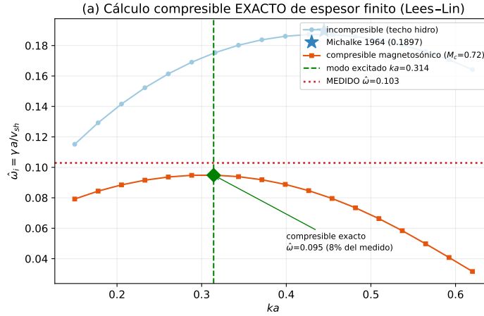
Figura 6.16: Cálculo compresible exacto de espesor finito (Lees-Lin), validado contra Michalke [21] en el límite incompresible. La curva magnetosónica pica en ka \simeq 0,32 con \hat{\omega} = 0,095 , justo en el modo excitado; el valor medido (0,103) coincide dentro del 8 %. [REV: los puntos estrella de incompresible y de michaelke no aparecen en la gráfica]
