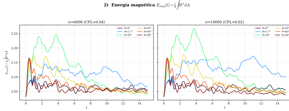
Figura 6.22: Campaña B: energía magnética E_{mag}(t) = \frac{1}{2} \int B^2 dA por ángulo; sus valles se acoplan con los picos de enstrofia.
