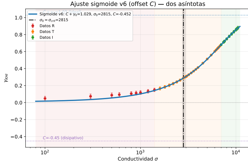
Figura 6.4: [REV: Ajuste sigmoide de la tasa de crecimiento efectiva \gamma_{KHI} en función de la conductividad eléctrica \sigma . Las bandas sombreadas indican los regímenes resistivo, transitorio e ideal. La línea vertical marca el valor crítico \sigma_{crit} , asociado al punto de inflexión del ajuste, mientras que la banda gris representa la incertidumbre ponderada en su estimación. Las líneas punteadas muestran las asíntotas del modelo: la asíntota superior C + \gamma_0 \simeq 1,03 , asociada al régimen casi ideal, y la asíntota inferior C \simeq -0,45 , que actúa como parámetro de offset del ajuste.] [REV: Yo evitaría llamar a C \simeq -0,45 "asíntota disipativa" como un dato físico fuerte, porque una tasa de crecimiento negativa puede sonar problemática si el lector espera crecimiento KHI.] Ajuste sigmoide con offset (v6) [REV: que es v6, versión 6? si es así es un dato irrelevante para el lector]. Las líneas punteadas marcan las dos asíntotas: C + \gamma_0 = 1,03 (ideal) y C = -0,45 (disipativo). Bandas: regímenes Resistivo/Transición/Ideal. La línea vertical es \sigma_0 = \sigma_{crit} y la banda gris el consenso ponderado.
