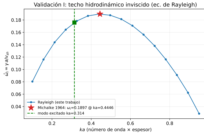
Figura 6.14: Validación del solver de autovalores. Tasa de crecimiento adimensional \hat{\omega}_i(ka) de la ecuación de Rayleigh (este trabajo) frente al valor de Michalke [21]. El cuadrado verde marca el modo excitado en las simulaciones.
