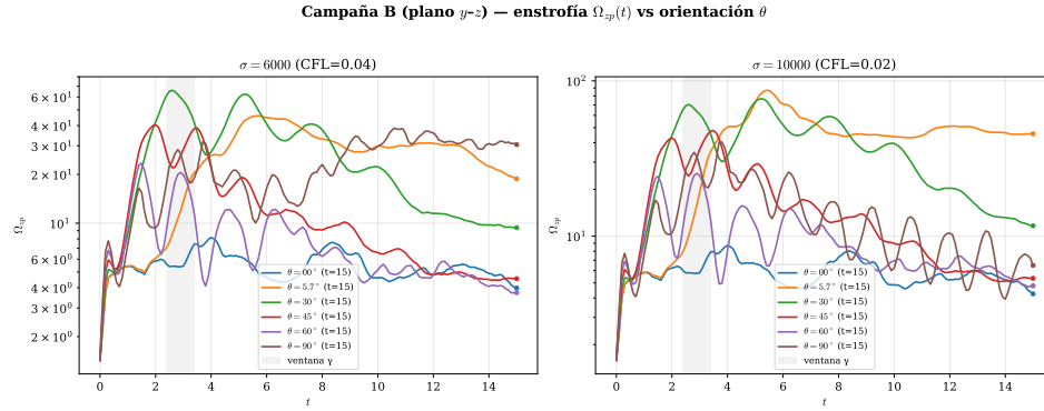
Figura 6.20: Campana B (orientación en el plano y - z ): \Omega_{zp}(t) por ángulo \theta , para ambas conductividades.
