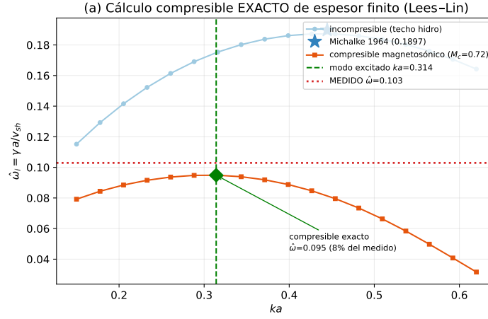
Figura 6.13: Cálculo compresible exacto de espesor finito (Lees-Lin), validado contra Michalke [17] en el límite incompresible. La curva magnetosónica pica en ka \simeq 0,32 con \hat{\omega} = 0,095 , justo en el modo excitado; el valor medido (0,103) coincide dentro del 8 %.
