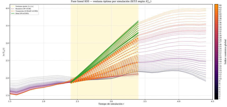
Figura 6.3: Extracción de \gamma_{KHI} : \ln \Omega_{zp}(t) para las 44 simulaciones (color = índice canónico, conductividad creciente del oscuro al naranja) con el ajuste lineal en la ventana sombreada [2, 4, 3, 4] . El estilo de cada recta codifica la calidad del ajuste por régimen: resistivo (punteado, R^2_{fija} < 0,90 ), transición (discontinuo, 0,90 \leq R^2_{fija} < 0,995 ) e ideal (continuo, R^2_{fija} \geq 0,995 ). La pendiente de cada recta es 2\gamma_{KHI} .
