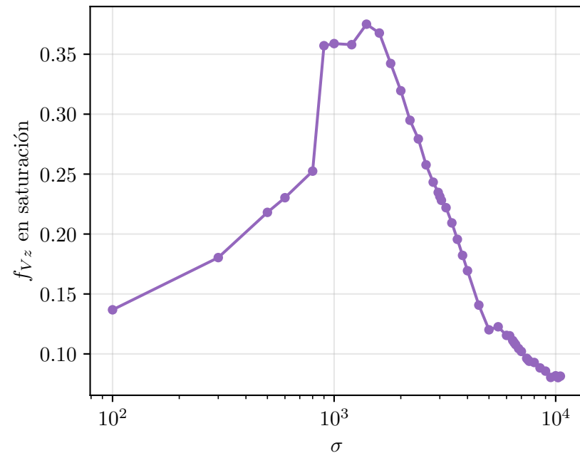
(a) Fracción de enstrofia fuera del plano
