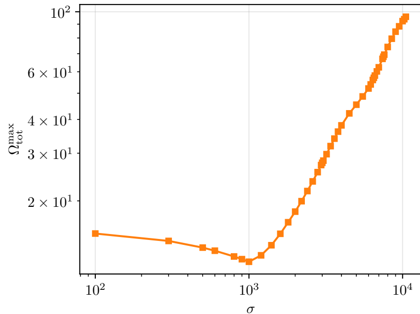
(b) Enstrofia total máxima (vórtices)
