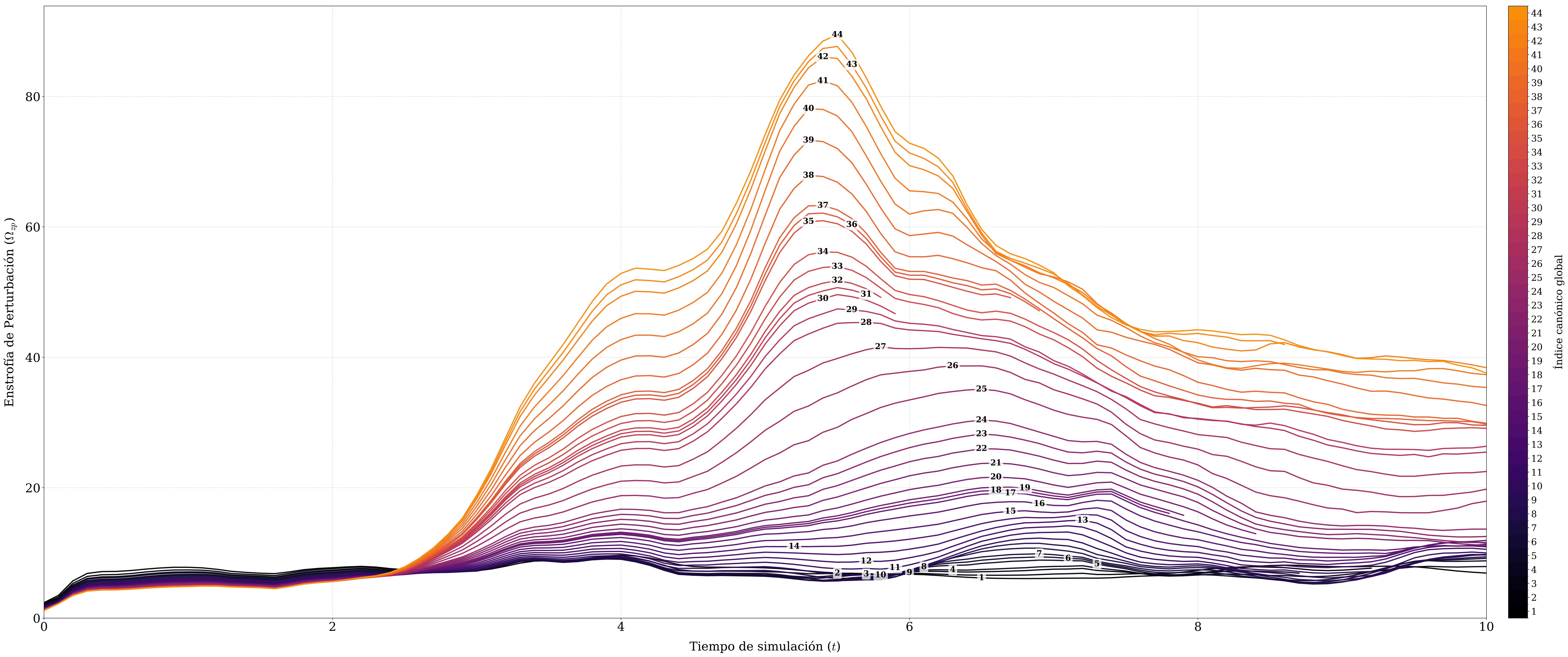
RRMHD-KHI: Enstrofía de Perturbación (supervivencia t > 3.0 , anotación t \in [5.0, 9.0] )
