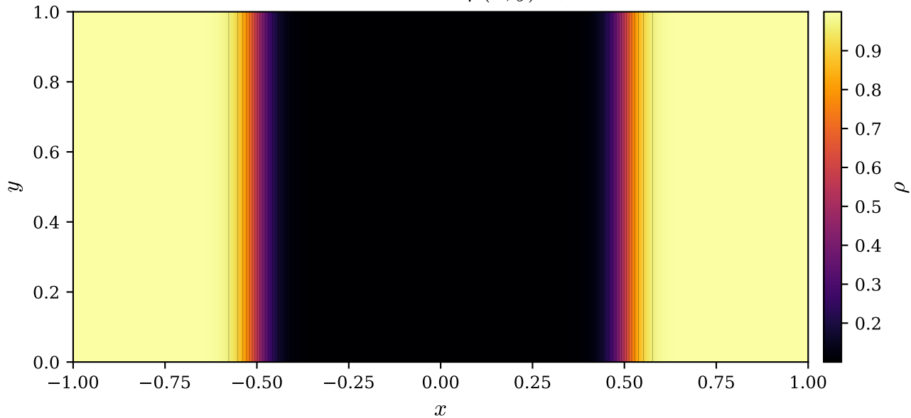
Densidad inicial \rho(x, y) ( t = 0 )
