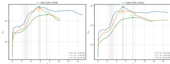
Campaña A — enstrofia \Omega_{sp}(t) vs intensidad B_0
