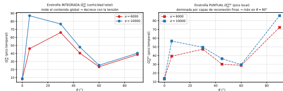
Campaña B: dos observables de enstrofia vs \theta — la "paradoja \theta = 90^\circ " es del observable puntual
