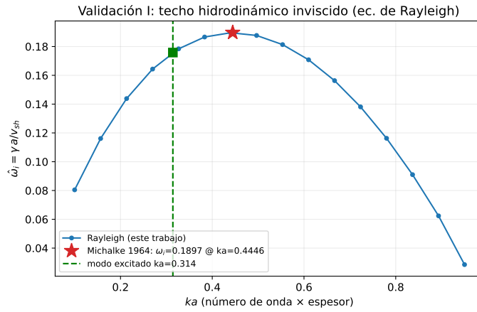
Figura 6.14: Validación del solver de autovalores. Tasa de crecimiento adimensional \hat{\omega}_i(ka) de la ecuación de Rayleigh (este trabajo) frente al valor de Michalke [22]. El cuadrado verde marca el modo excitado en las simulaciones.
