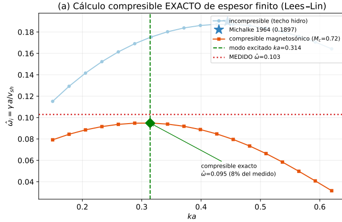
Figura 6.16: Cálculo compresible exacto de espesor finito (Lees-Lin), validado contra Michalke [22] en el límite incompresible. La curva magnetosónica pica en ka \simeq 0,32 con \hat{\omega} = 0,095 , justo en el modo excitado; el valor medido (0,103) coincide dentro del 8%. [REV: los puntos estrella de incompresible y de michaelke no aparecen en la gráfica]
