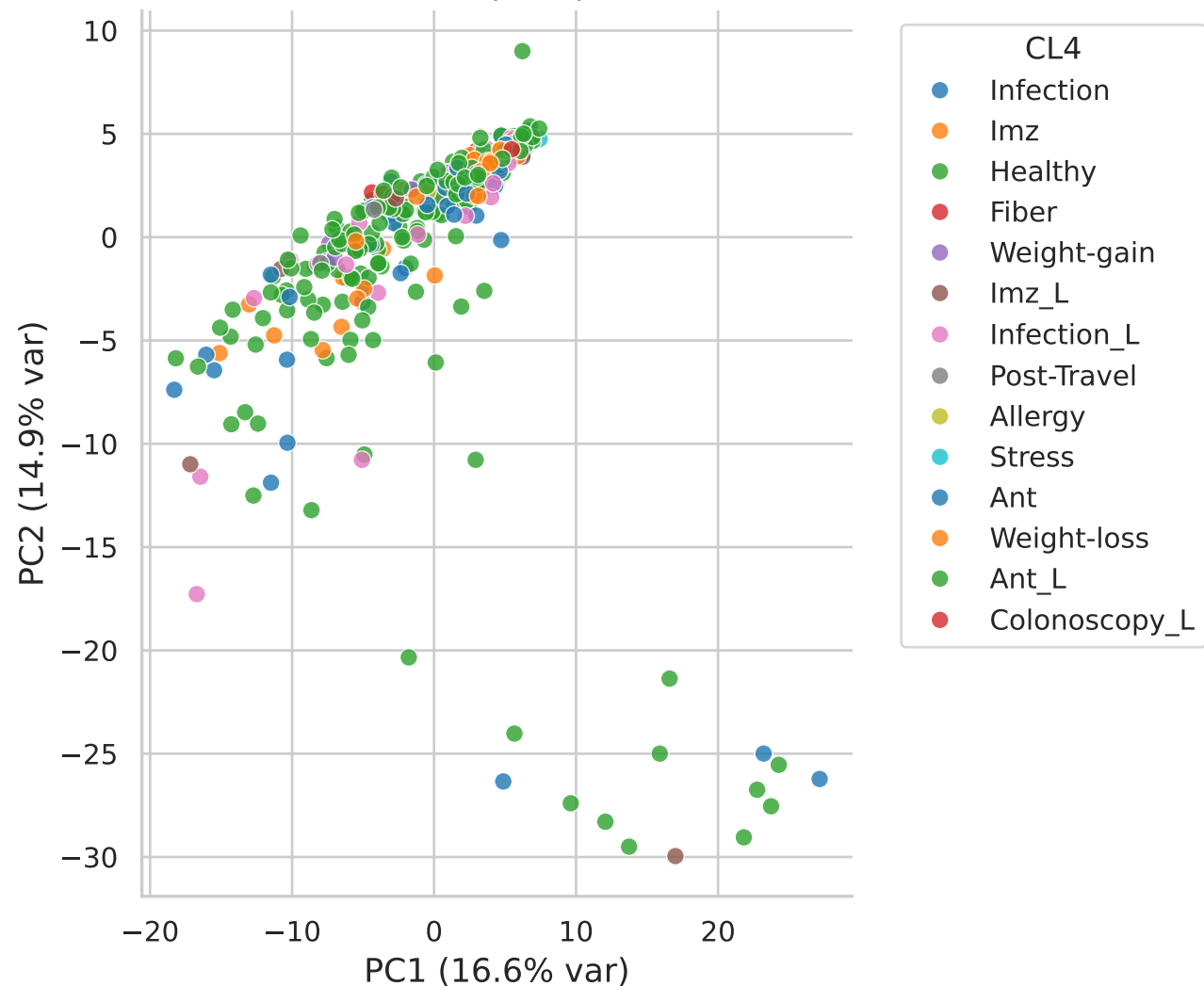
PCA (Skin)
