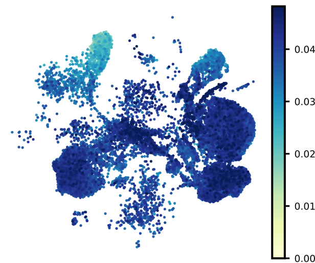
NFE2L1
