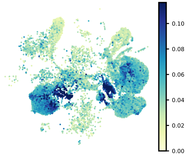
RELB
