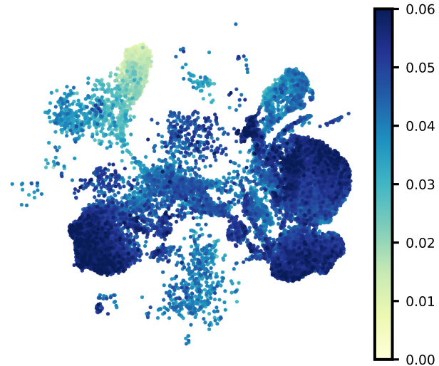
NFIC
