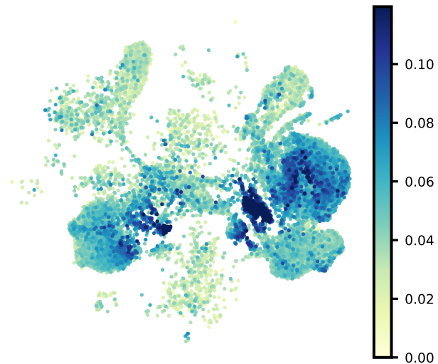
NFIC
