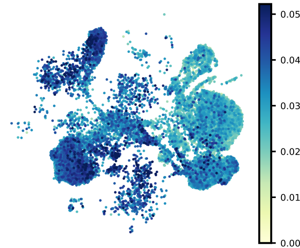
EP300
