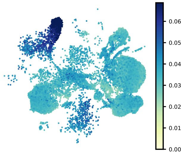
GATAD1
