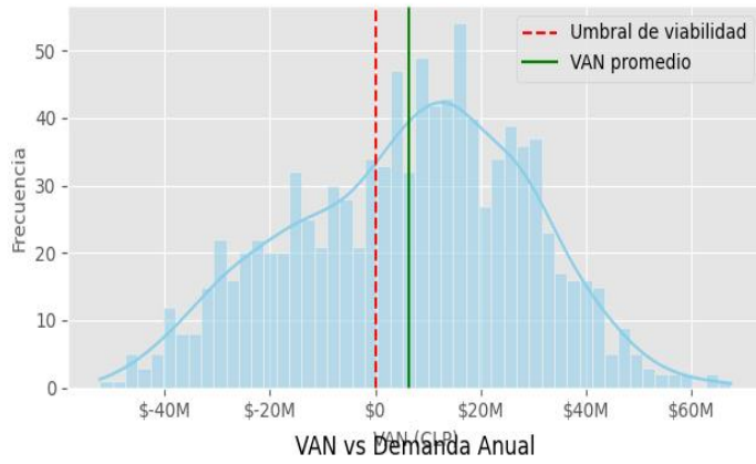
Distribución del Valor Actual Neto (VAN)
