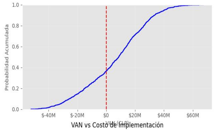
Probabilidad Acumulada del VAN
