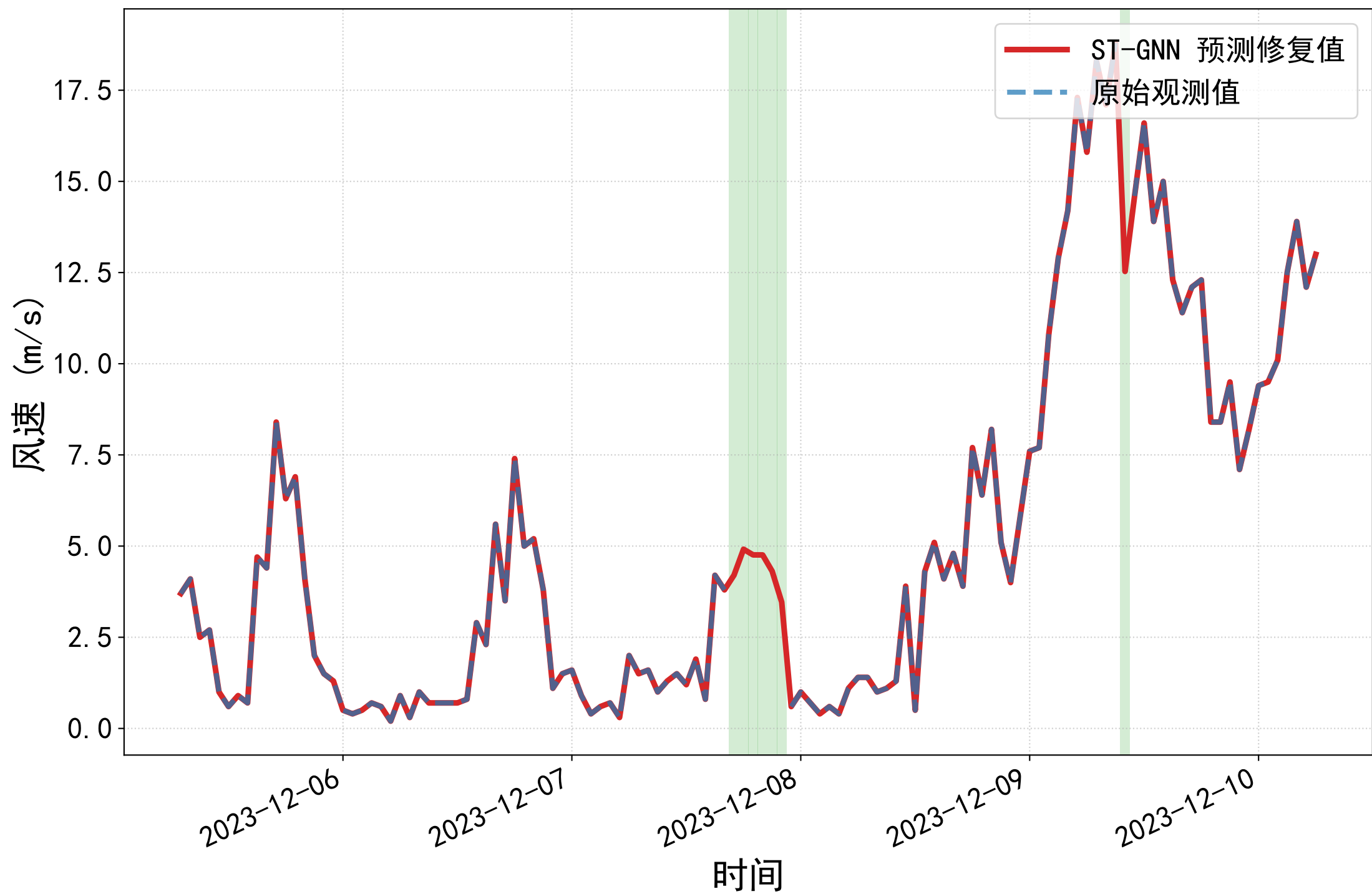
图2 典型机组短期风速修复时序图 (节点ID: id_53662)
