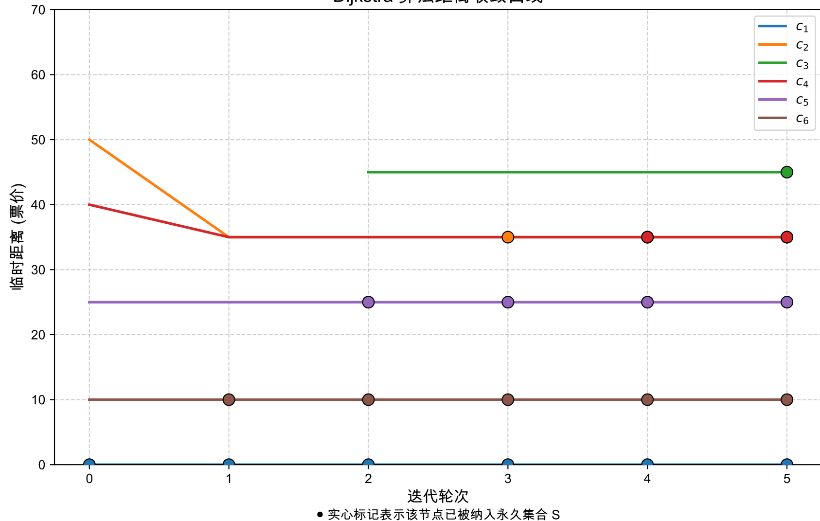
Dijkstra 算法距离收敛曲线
