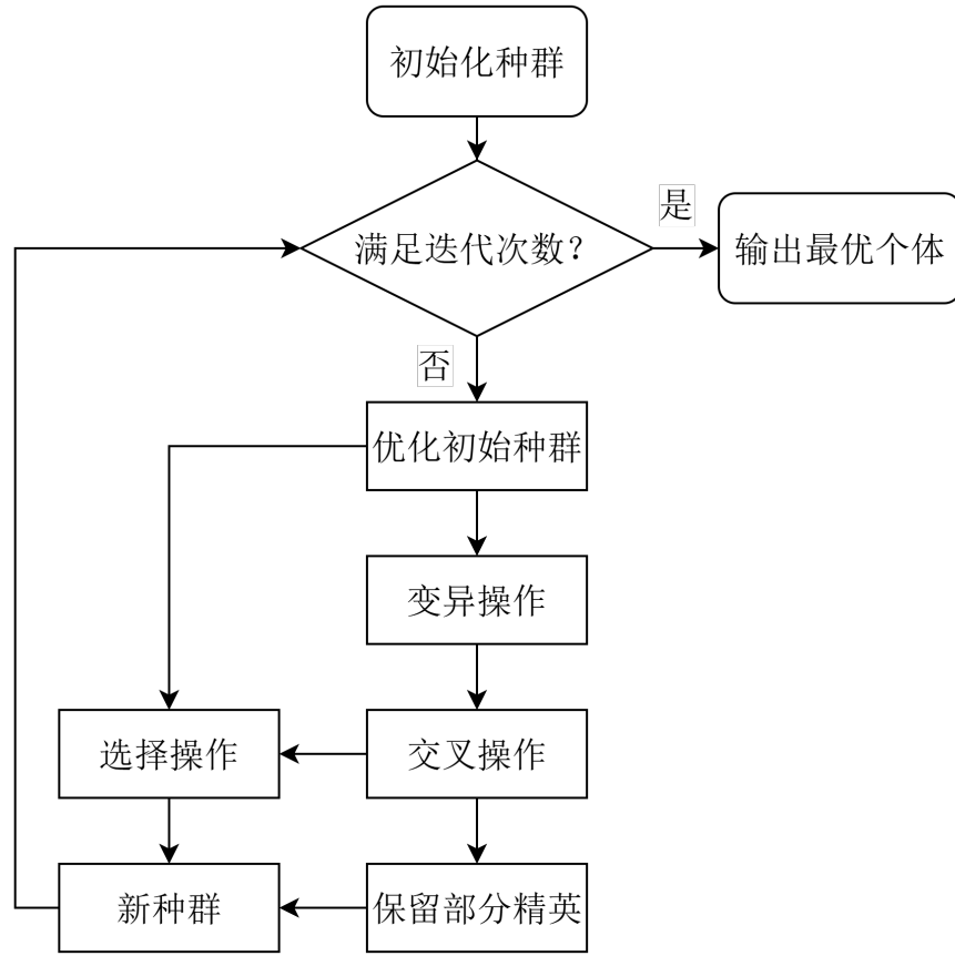
图 11: 差分进化算法流程图
