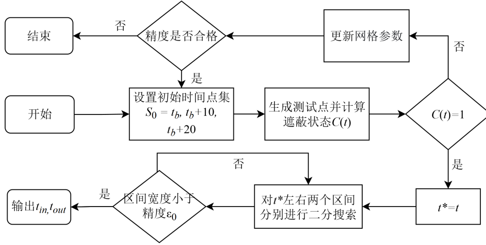
图 9: 问题一算法总体流程图
