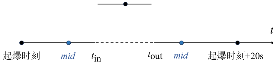
图 10: 二分查找法示意图
