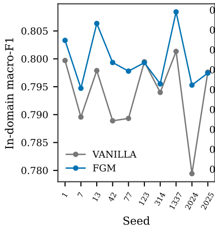
Ben-Sarc
