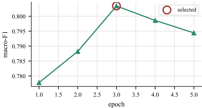
Validation macro-F1
