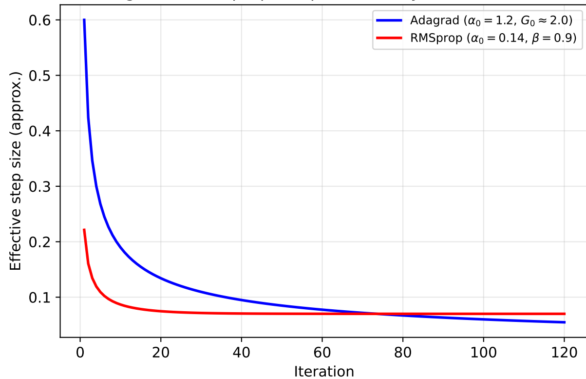
Adagrad vs RMSprop: Step Size Decay (Benchmark B)
