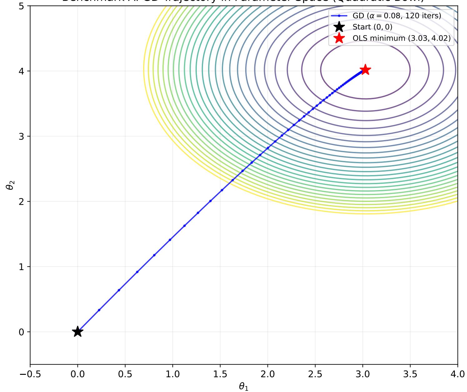
Benchmark A: GD Trajectory in Parameter Space (Quadratic Bowl)
