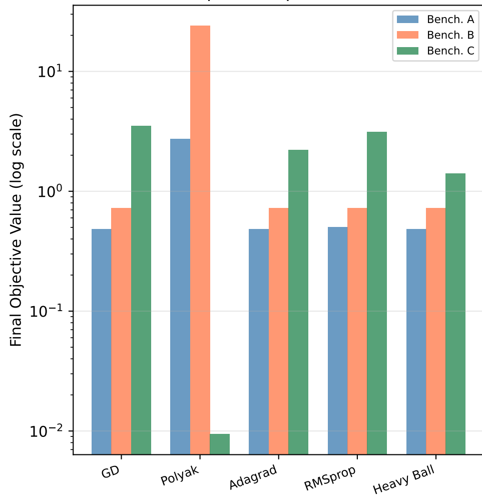
Q1: Adaptive Step-Size Methods
