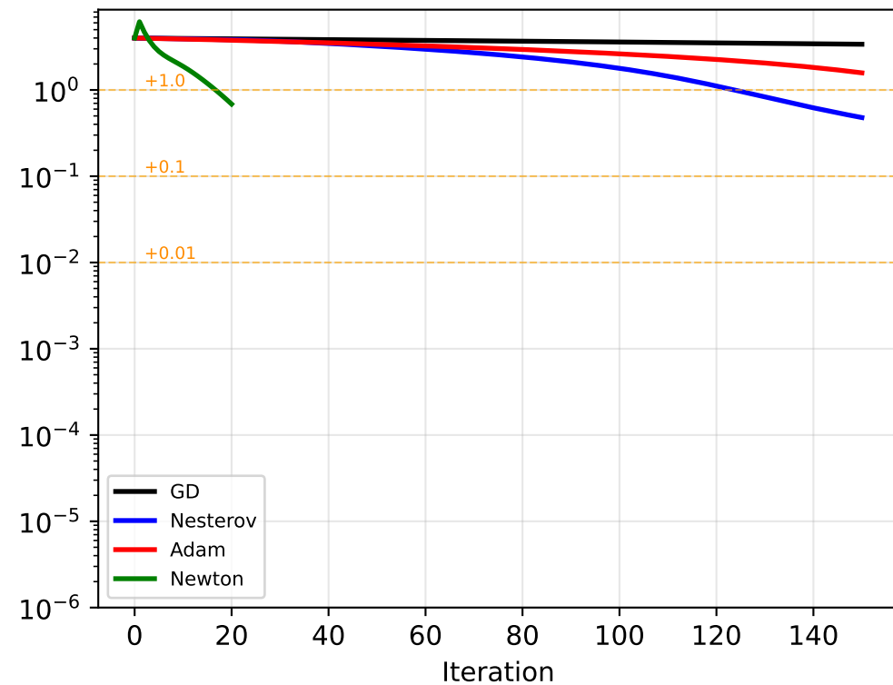
Benchmark C (Rosenbrock)
