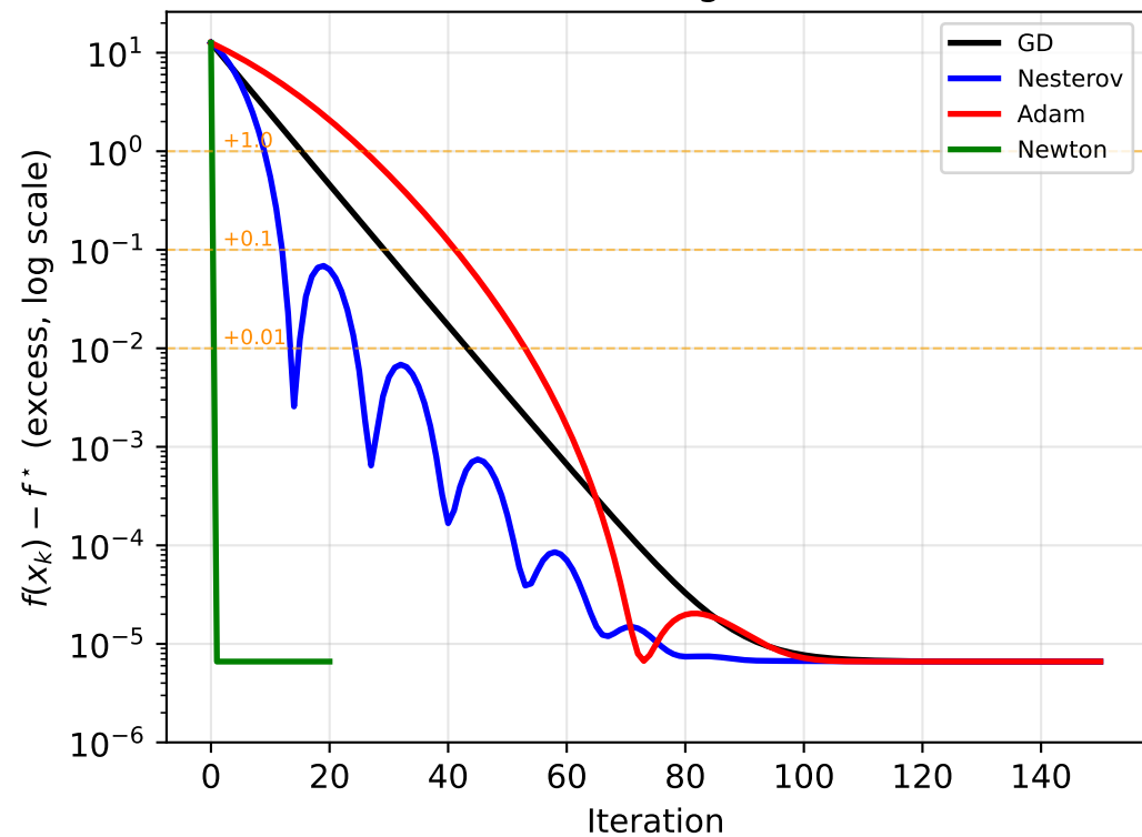
Benchmark A (LinReg)
