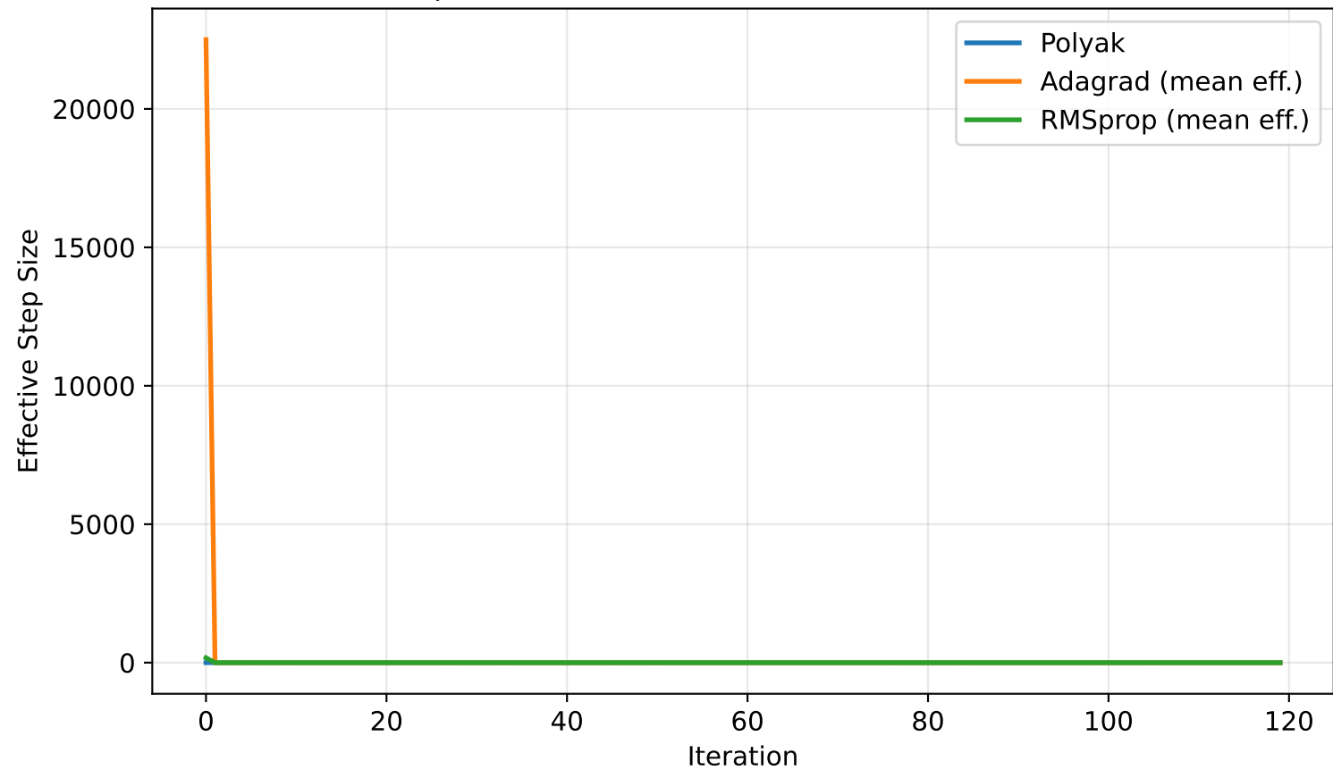
Q1: Step-Size Evolution — Benchmark C (Rosenbrock)
