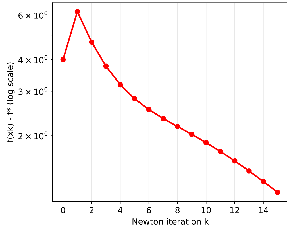
Benchmark C (Rosenbrock)
