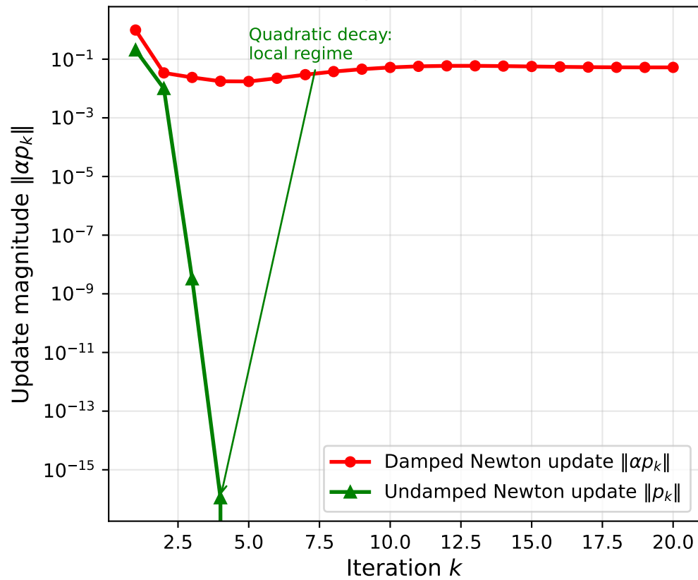
Newton Update Magnitude
