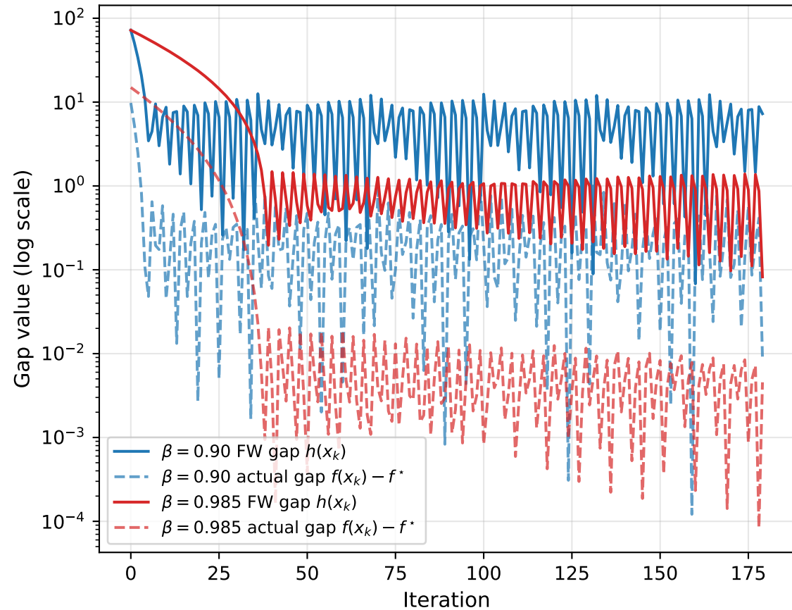
FW gap h(x_k) vs actual gap f(x_k) - f^* (interior case)
