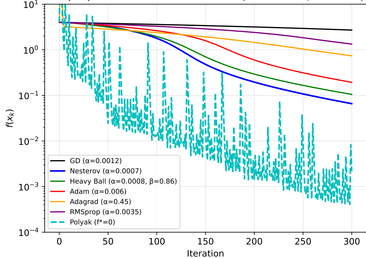
All Q1-Q2 methods on Benchmark C (Rosenbrock, 300 iters)
